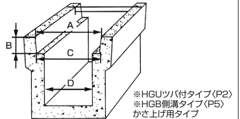
③ ロングU字溝 (工場生産品)
