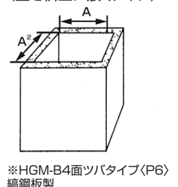
⑦ 改良ます (蓋を柵上に敷くタイプ)
