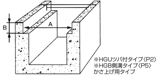
② 側溝 (蓋を溝中にはめ込むタイプ)
