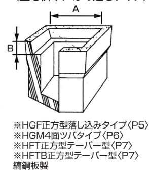
⑥ ためます (蓋を柵中にはめ込むタイプ)
